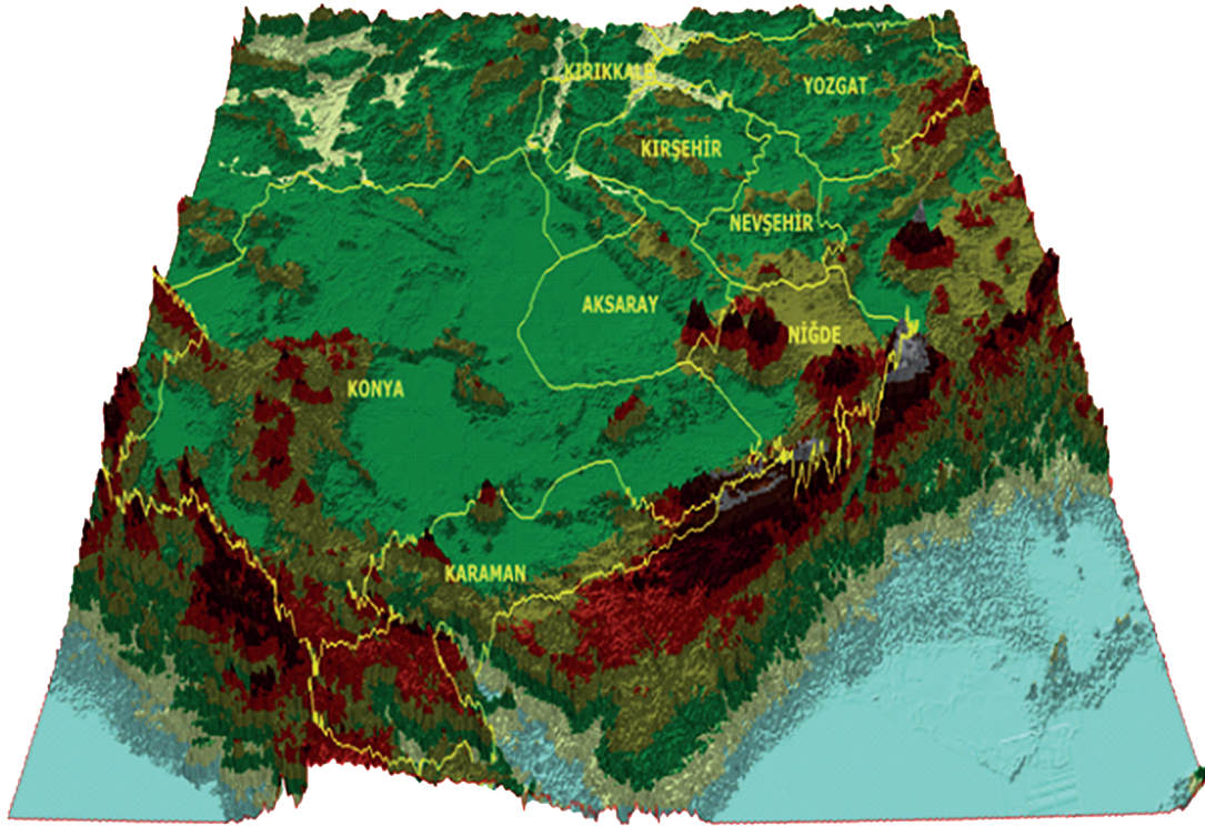
Şekil 21 KOP Bölgesi Havzalarının 3 Boyutlu Görüntüsü
