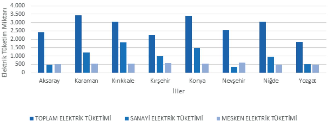
Şekil 40 KOP Bölgesi İllerinin Elektrik Tüketim Miktarı (2018)
