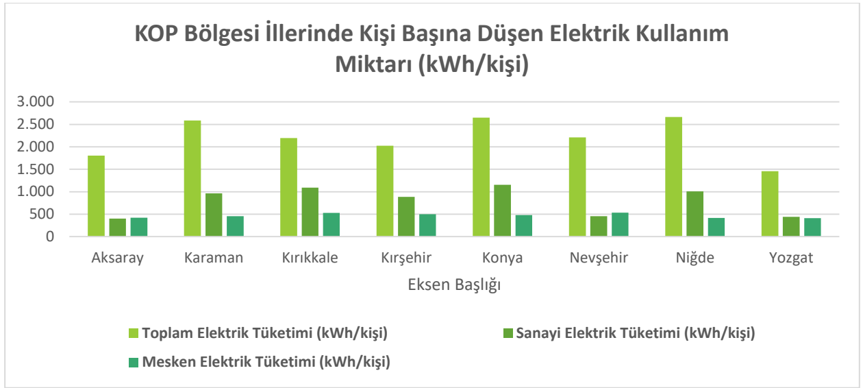
Şekil 43 KOP Bölgesi İllerinin Elektrik Tüketim Miktarı (2015)
