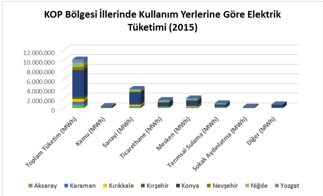
Şekil 42 KOP Bölgesi İlleri Kullanım Yerlerine Göre Elektrik Tüketimi (2015)
