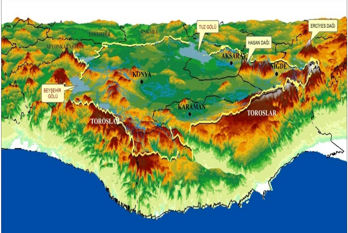
Şekil 19 KOP Bölgesi Kapalı Havzasının 3 Boyutlu Görüntüsü, (Akdeniz'e Kapalı Sıra Dağlar)
