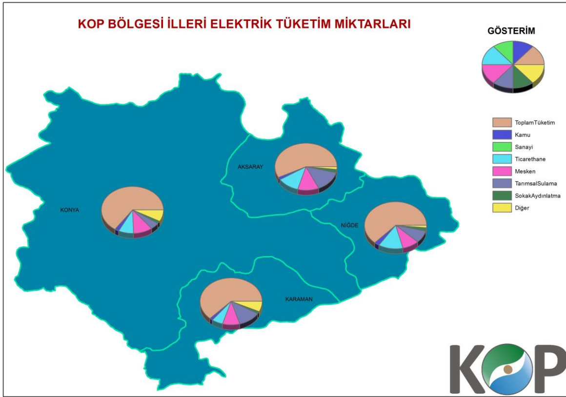
Şekil 36 KOP Bölgesi İllerinin Elektrik Tüketim Miktarları (2014)
